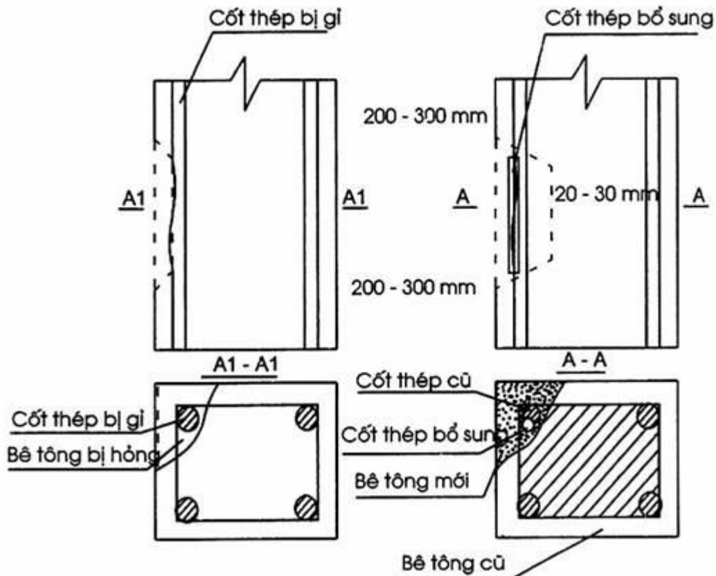
Hình A.1 – Bổ sung cốt thép bị hư hỏng cục bộ nhưng không mở rộng tiết diện kết cấu A.3.3.3. Gia cố bằng thép hình hoặc thép tròn có mở rộng tiết diện kết cấu
