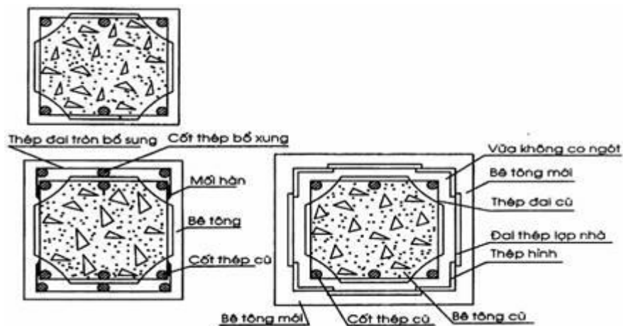
Hình A.2 – Gia cố mở rộng tiết diện kết cấu
