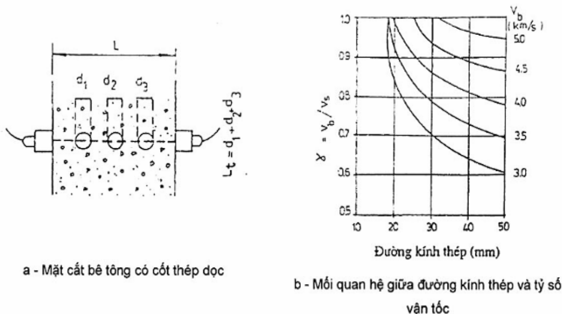
Hình 5 - Ảnh hưởng của cốt thép đến vận tốc xung khi thép nằm vuông góc với đường truyền xung
