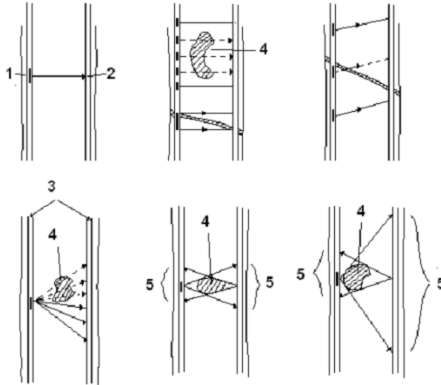
Hình C.5 - Biểu đồ vận tốc và năng lượng truyền xung siêu âm
